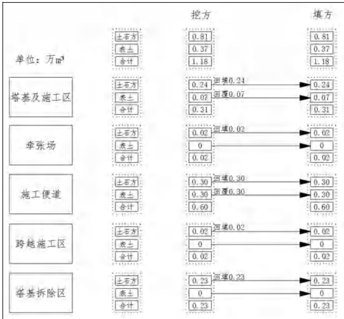
图 2-4 总土石方流向框图
